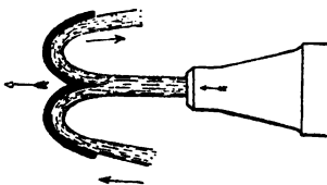
Fig. 58. Schaufelform des Peltonrads.
